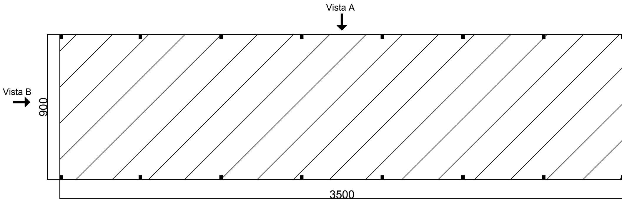
Planta Baixa A = 315,00 m 2
